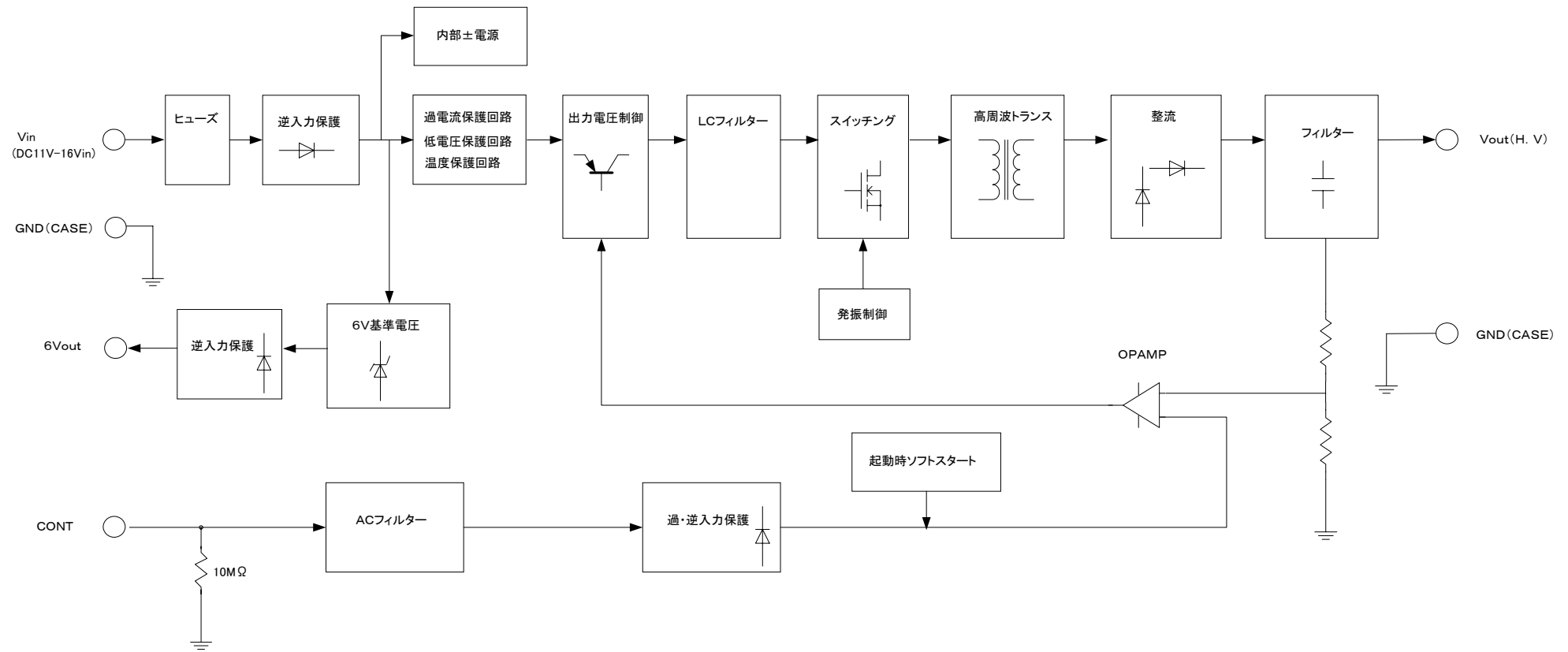
(中)高圧電源機能ブロック図
