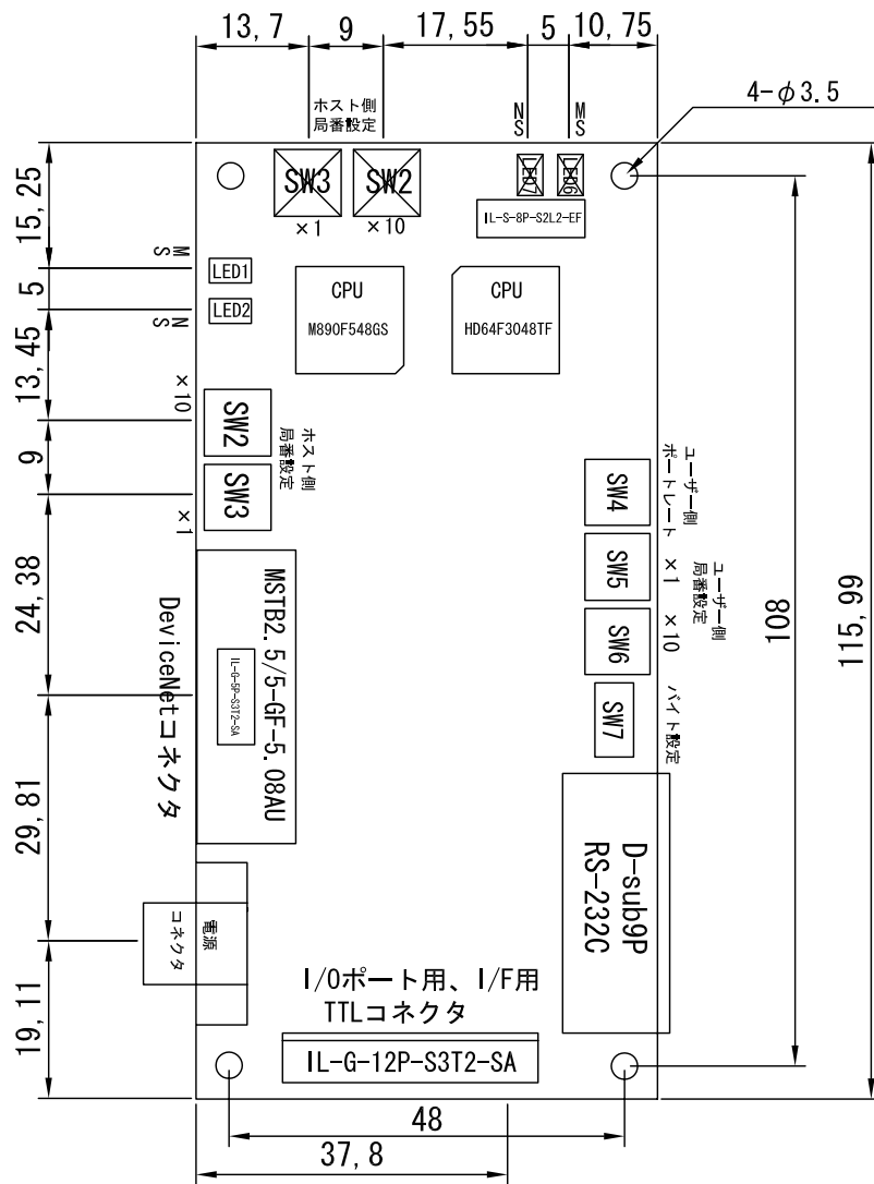
DNS-GW外形図 ×: 未実装です。
