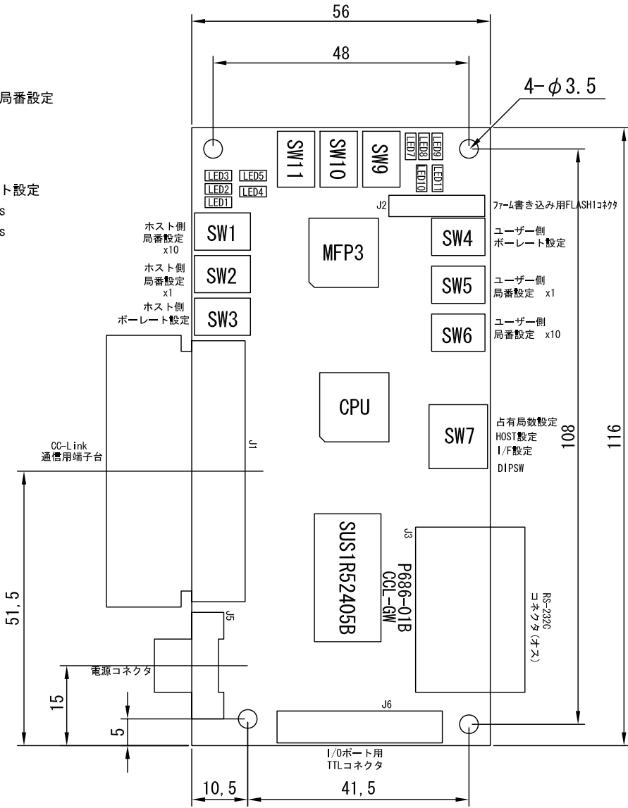
CCL-GW外形図
